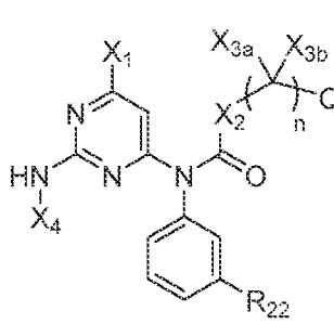
(XIa),
