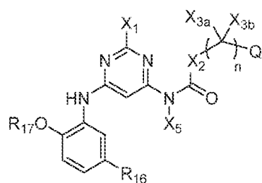
(VIIIa),
