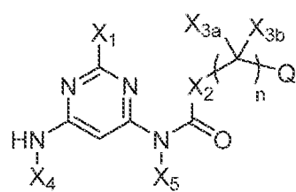
(Va),
