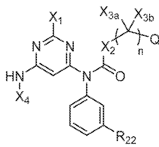
(XIa),
