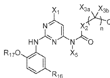
(VIIIa),
