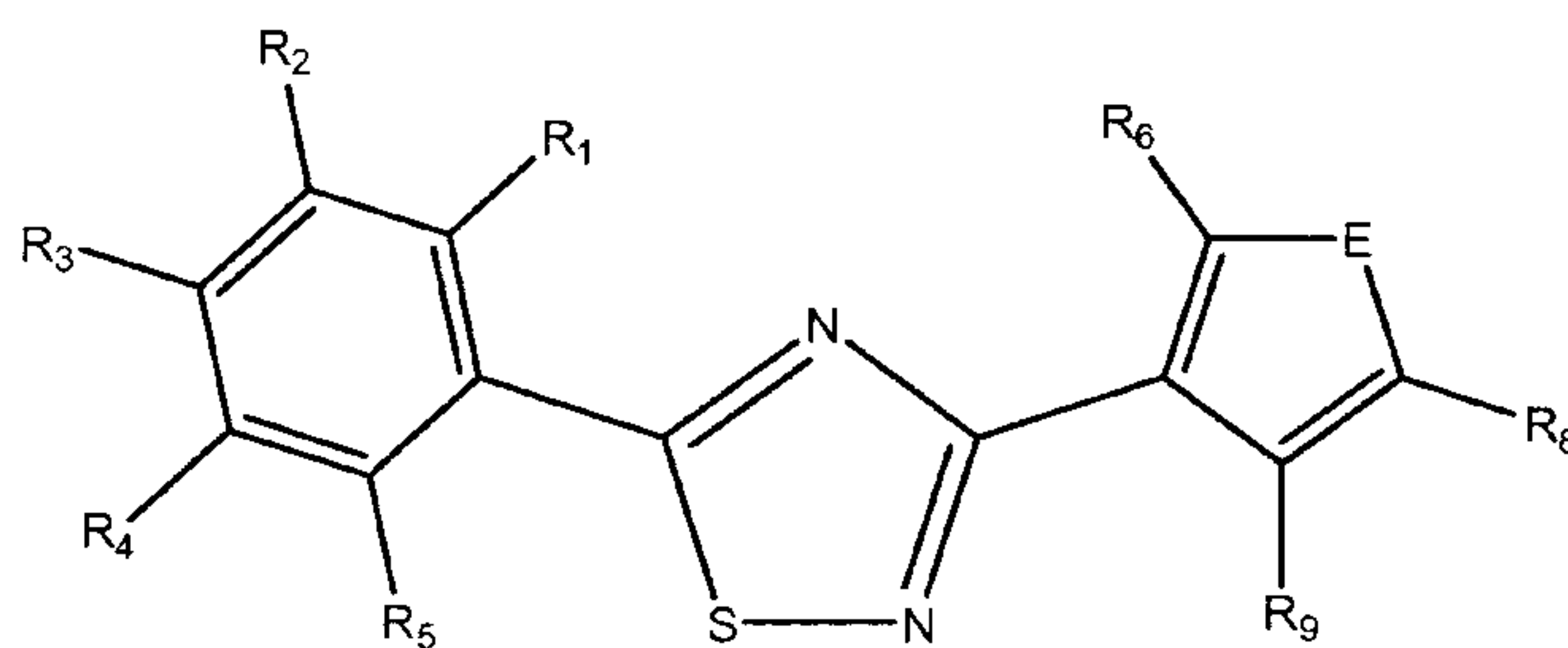
Formula VIIb
