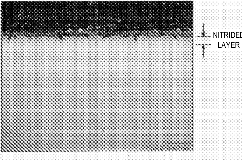
EXAMPLE (d) (NCF600 : W/ GRINDING AFTER 1000 TIMES NITRIDING TREATMENT)
