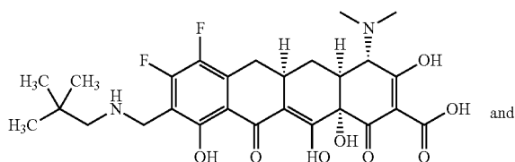
IVb
