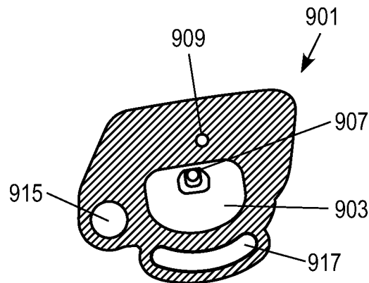
SECTION D-D FIG. 11
