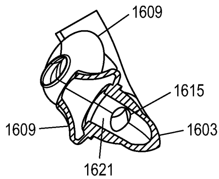
FIG. 19C SECTION G-G
