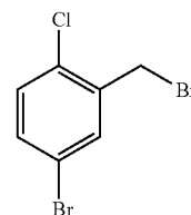
4-bromo-2-bromomethyl-1-chloro-benzene
