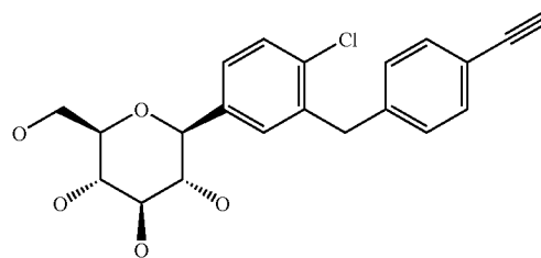
1-chloro-4-(β-D-glucopyranos-1-yl)-2-(4-ethynylbenzyl)-benzene
