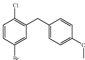
4-bromo-1-chloro-2-(4-methoxy-benzyl)-benzene
