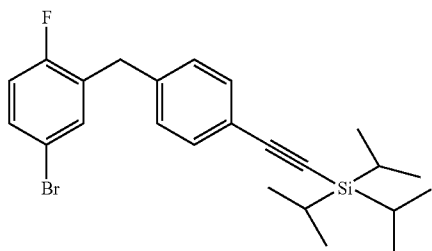
[4-(5-bromo-2-fluoro-benzyl)-phenylethynyl]-triisopropyl-silane
