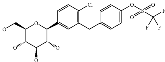
1-chloro-4-(β-D-glucopyranos-1-yl)-2-[4-(trifluoromethylsulphonyloxy)-benzyl]-benzene
