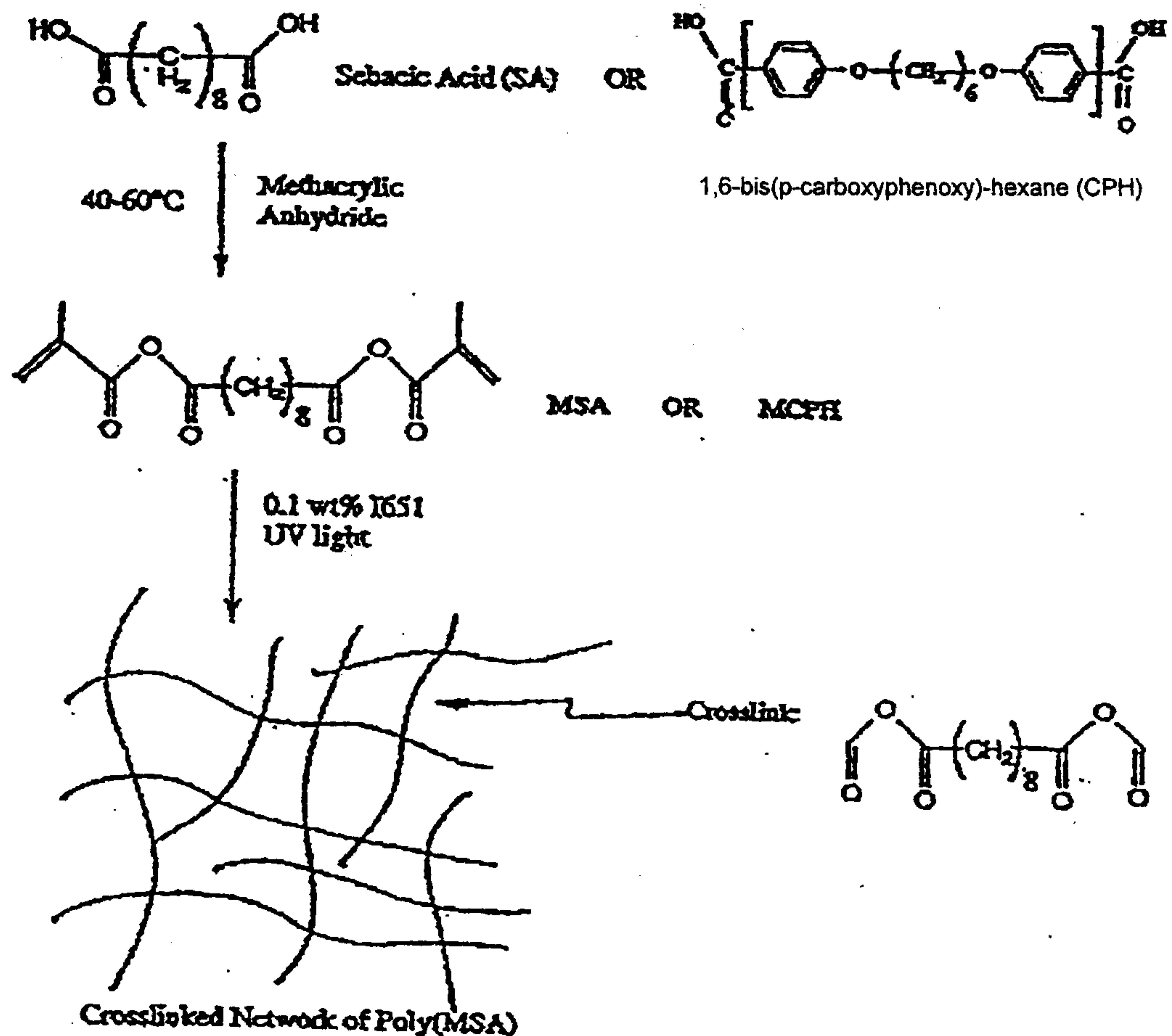
Scheme I:
