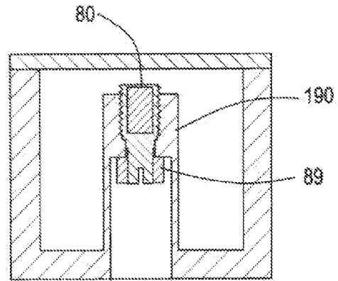
SECTION A-A FIG. 11B
