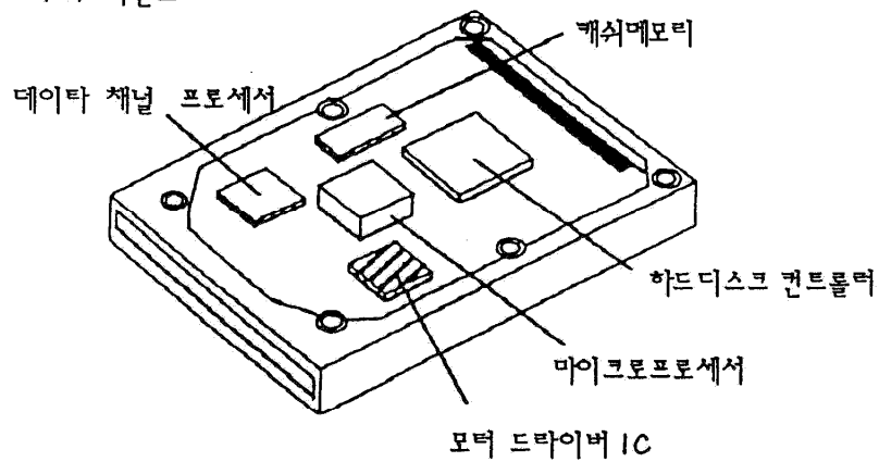
(b) 하면도
