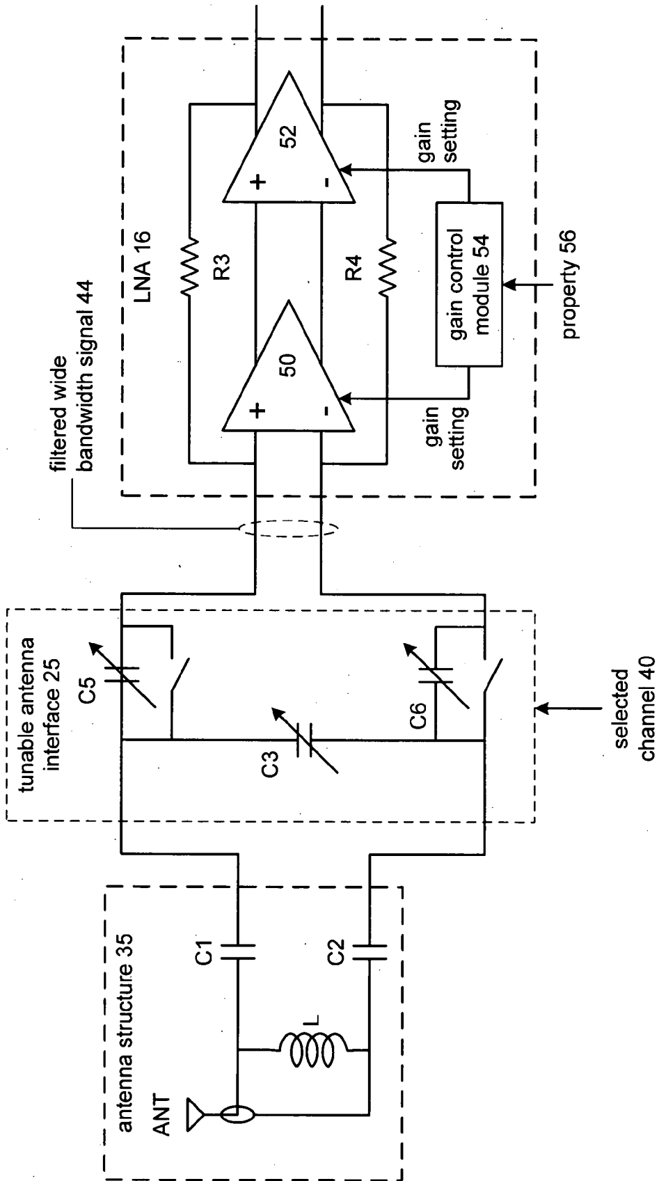
FIG. 3 front-end 15
