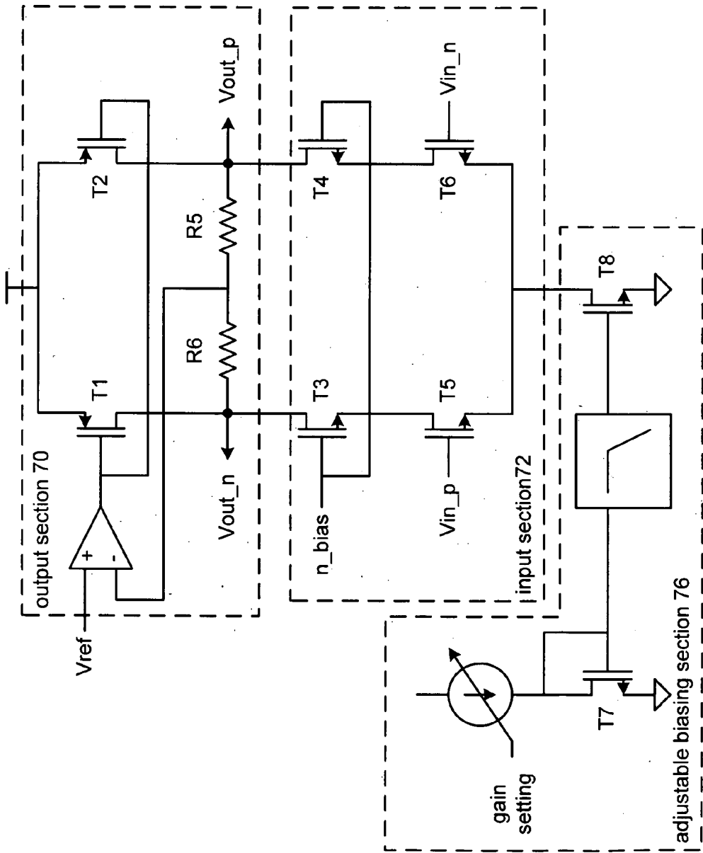
FIG. 4 amplifier 50 or 52
