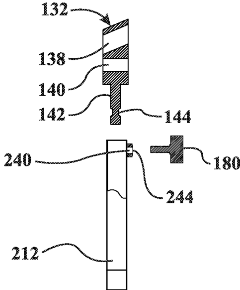
Section A-A FIG. 52
