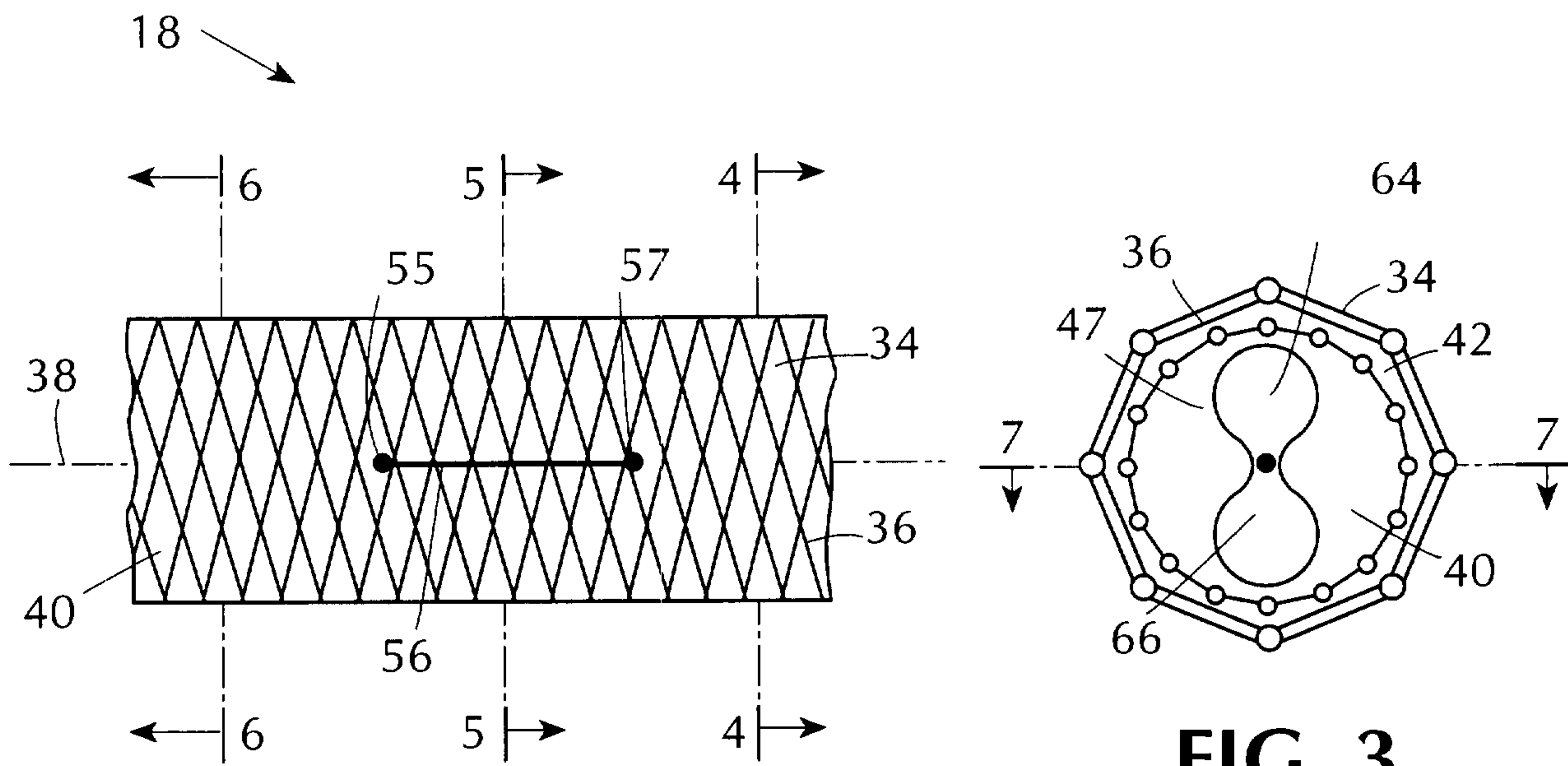
FIG. 2
