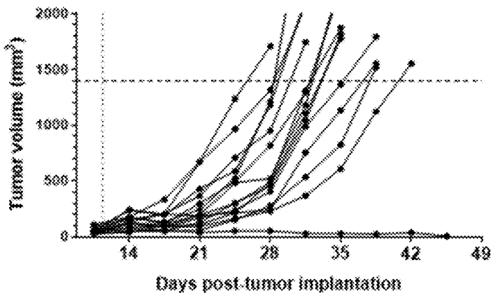
1e7 Cop.Luc-GFP.A34-K151E (IT dosing on D10)
