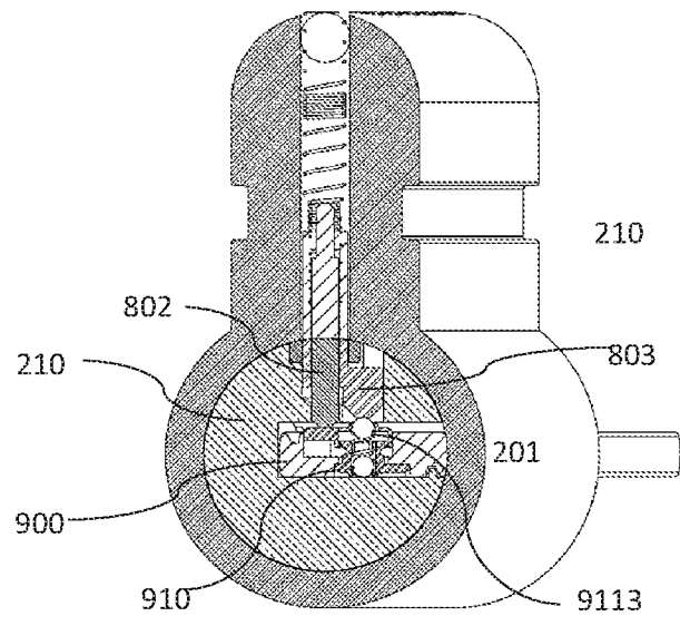
FIG. 10C
