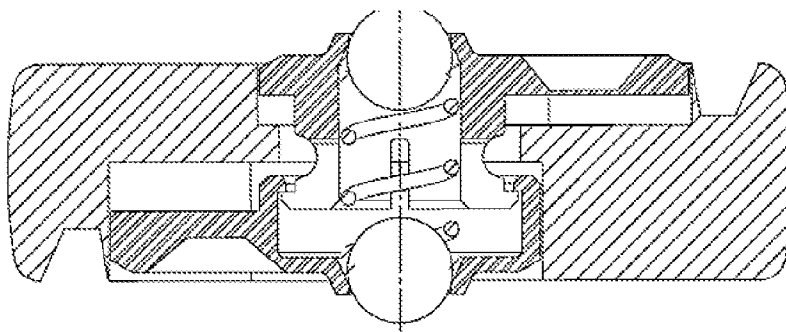
FIG. 11B
