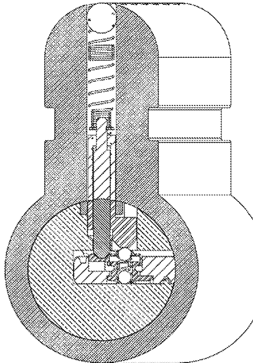
FIG. 11C
