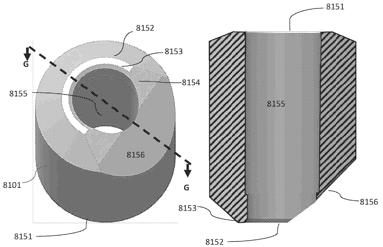
FIG. 14A
