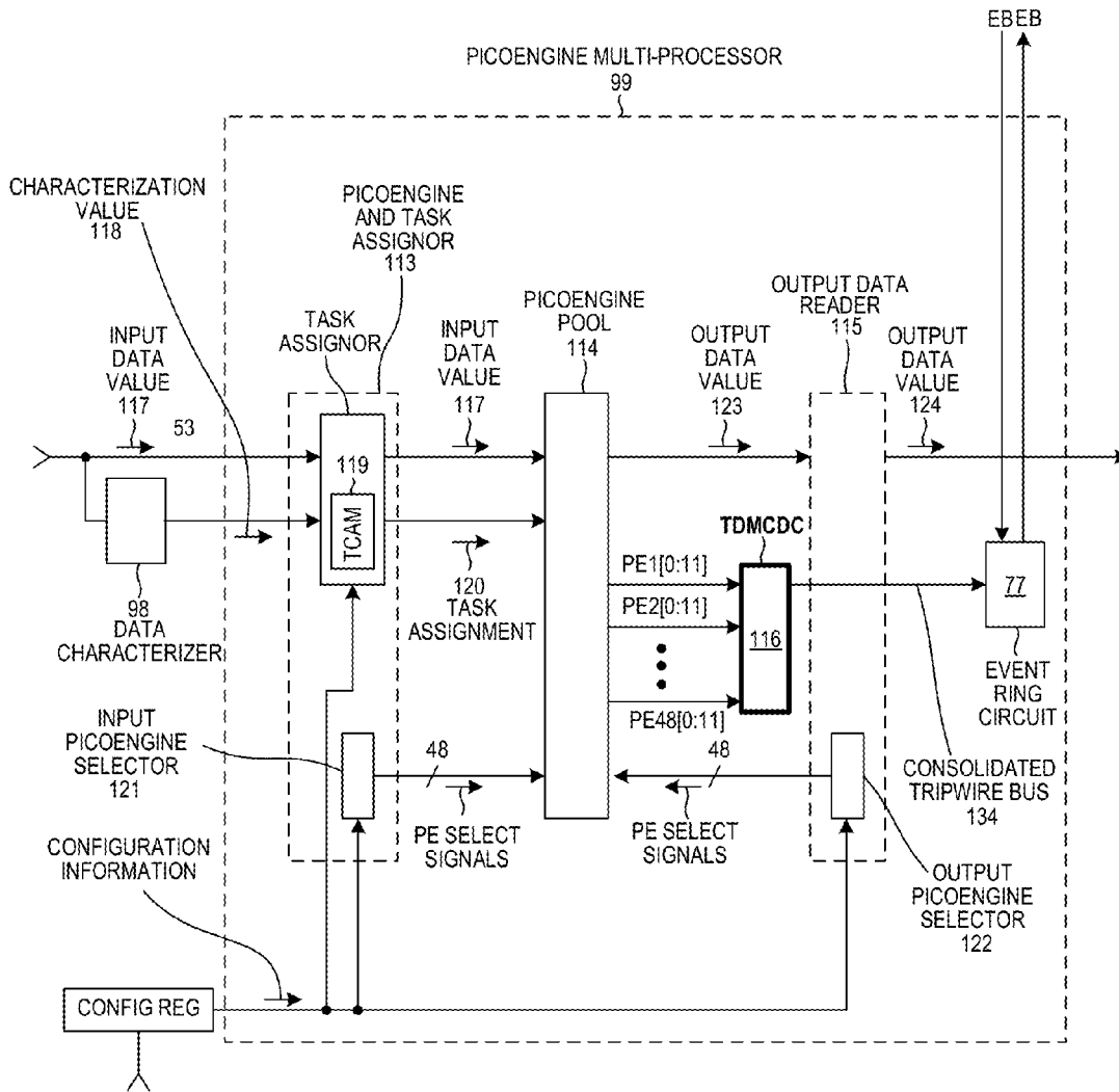
PICOENGINE MULTI-PROCESSOR FIG. 9
