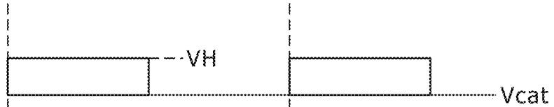
FIG. 32A DUTY50%
