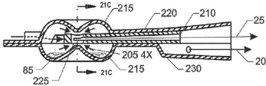
Section 21B-21B
