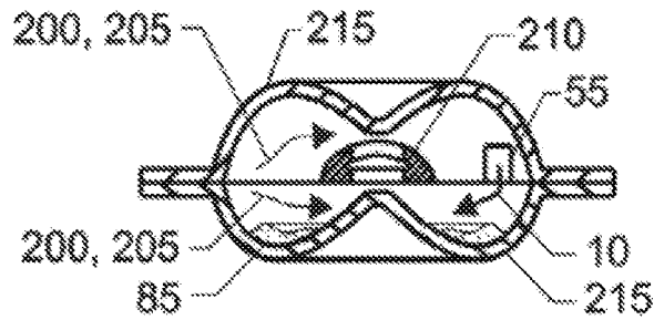
Section 21C-21C
