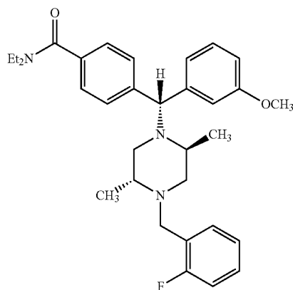
4-((alpha-R)-alpha-((2S,5R)-2,5-Dimethyl-4-(2-fluorobenzyl)-1-piperazinyl)-3-methoxybenzyl)-N,N-diethylbenzamide
