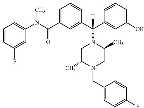
3-((R)-((2S,5R)-2,5-Dimethyl-4-(4-fluorobenzyl)-1-piperazinyl)-3-hydroxybenzyl)-N-(3-fluorophenyl)-N-methylbenzamide
