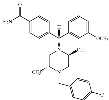
4-((alpha-R)-alpha-((2S,5R)-2,5-Dimethyl-4-(4-fluorobenzyl)-1-piperazinyl)-3-methoxybenzyl)-N,N-diethylbenzamide
