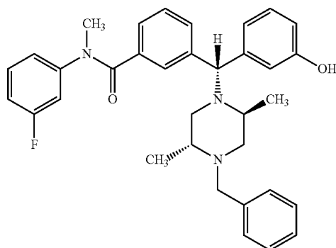
3-((R)-((2S,5R)-4-Benzyl-2,5-dimethyl-1-piperazinyl)-3-hydroxybenzyl)-N-(3-fluorophenyl)-N-methylbenzamide
