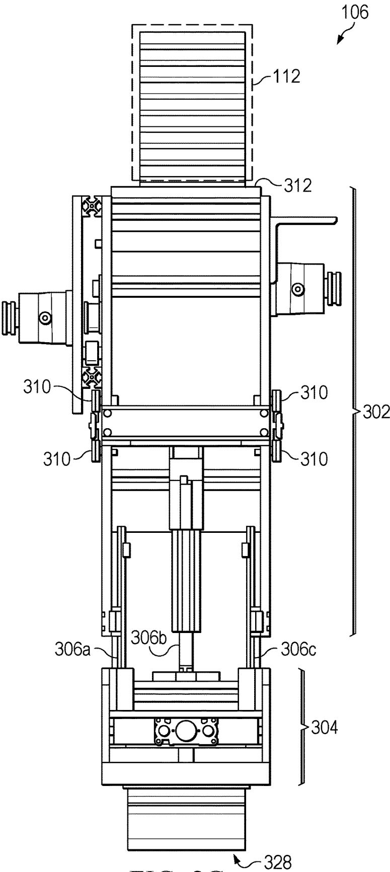
FIG. 3C
