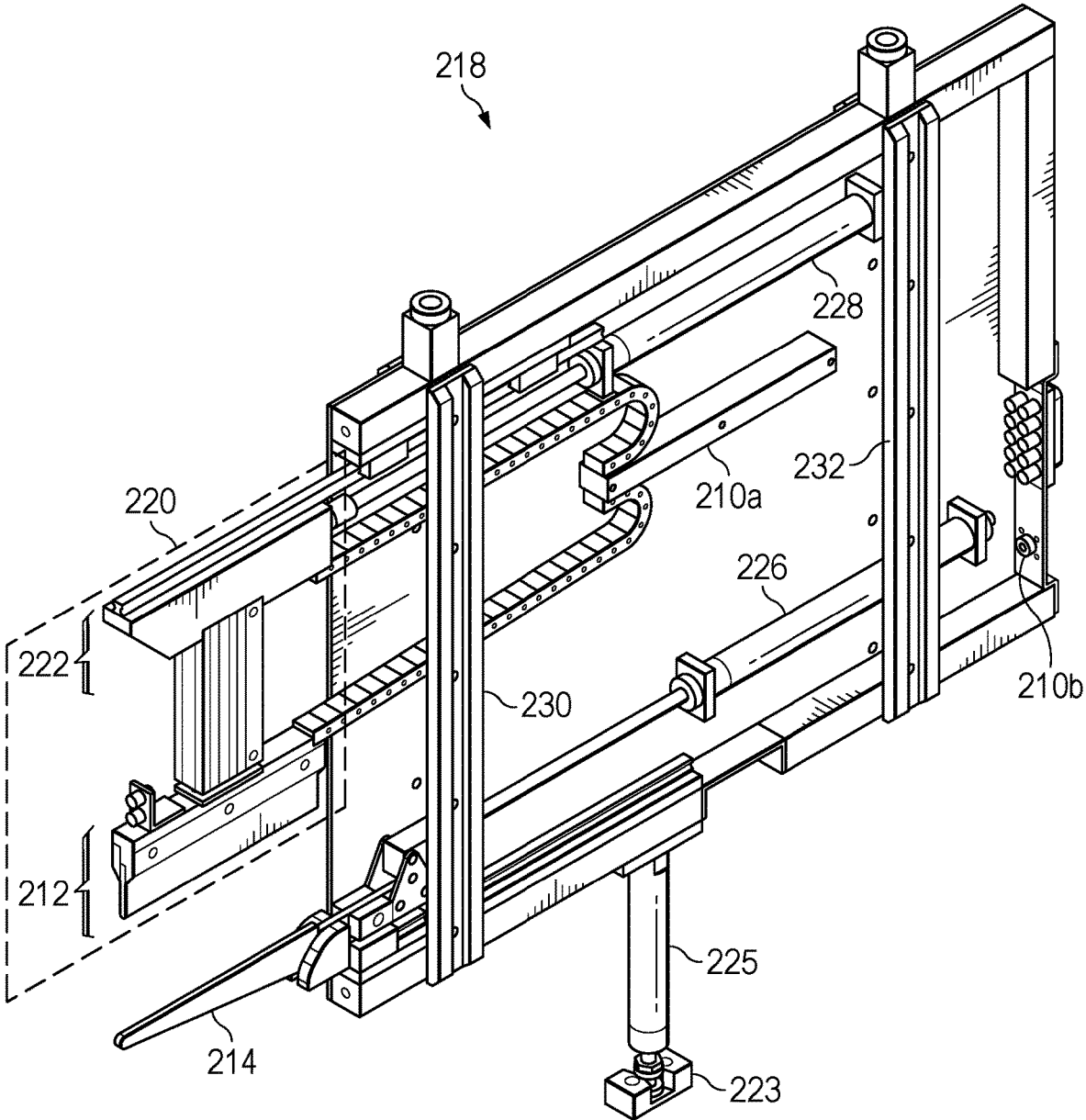
FIG. 2G
