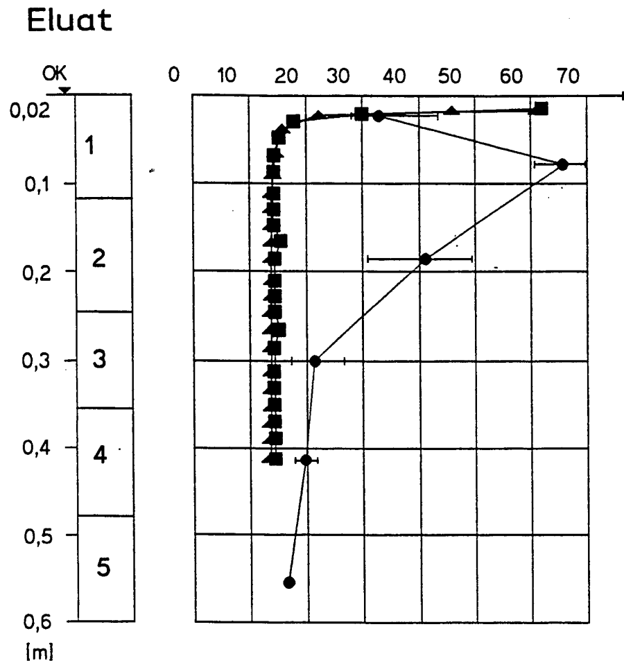
Abb. 2: Konzentrationen als Funktion der Eindringtiefe
