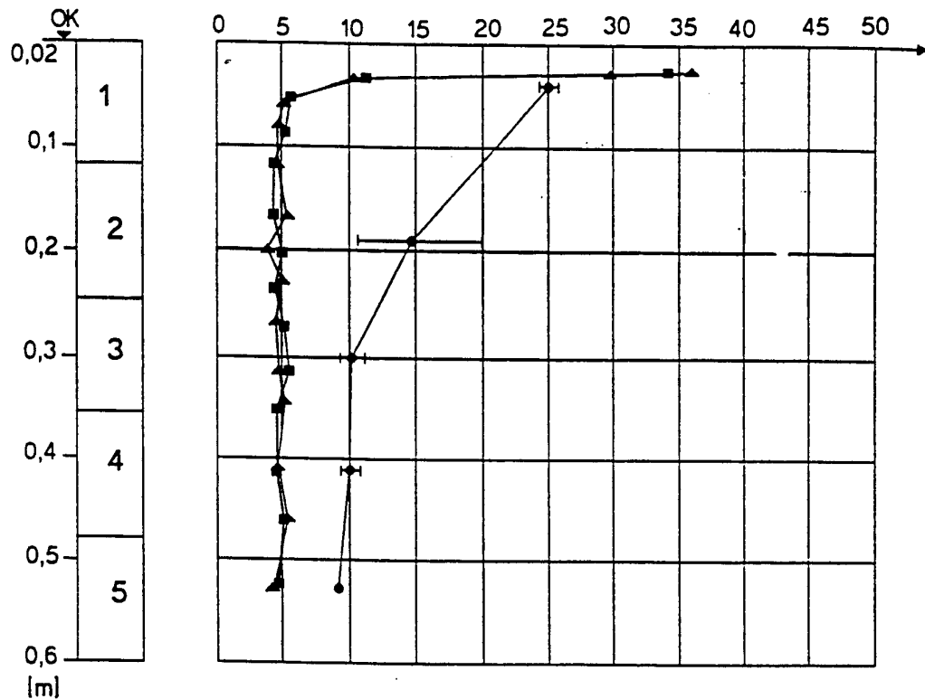
Abb. 6: Konzentrationen als Funktion der Eindringtiefe
