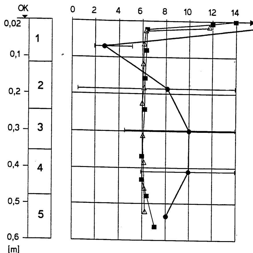
Abb. 5: Konzentrationen als Funktion der Eindringtiefe
