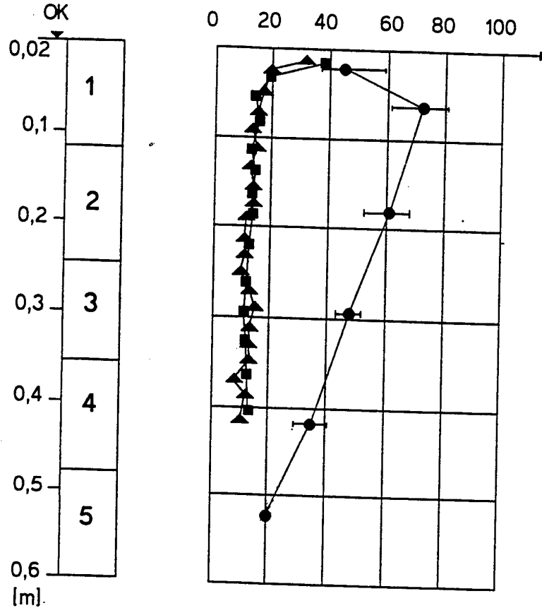
Abb. 4: Konzentrationen als Funktion der Eindringtiefe
