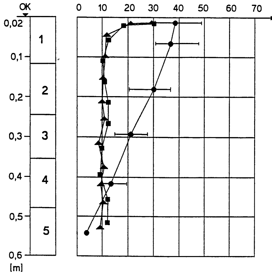
Abb. 3: Konzentrationen als Funktion der Eindringtiefe
