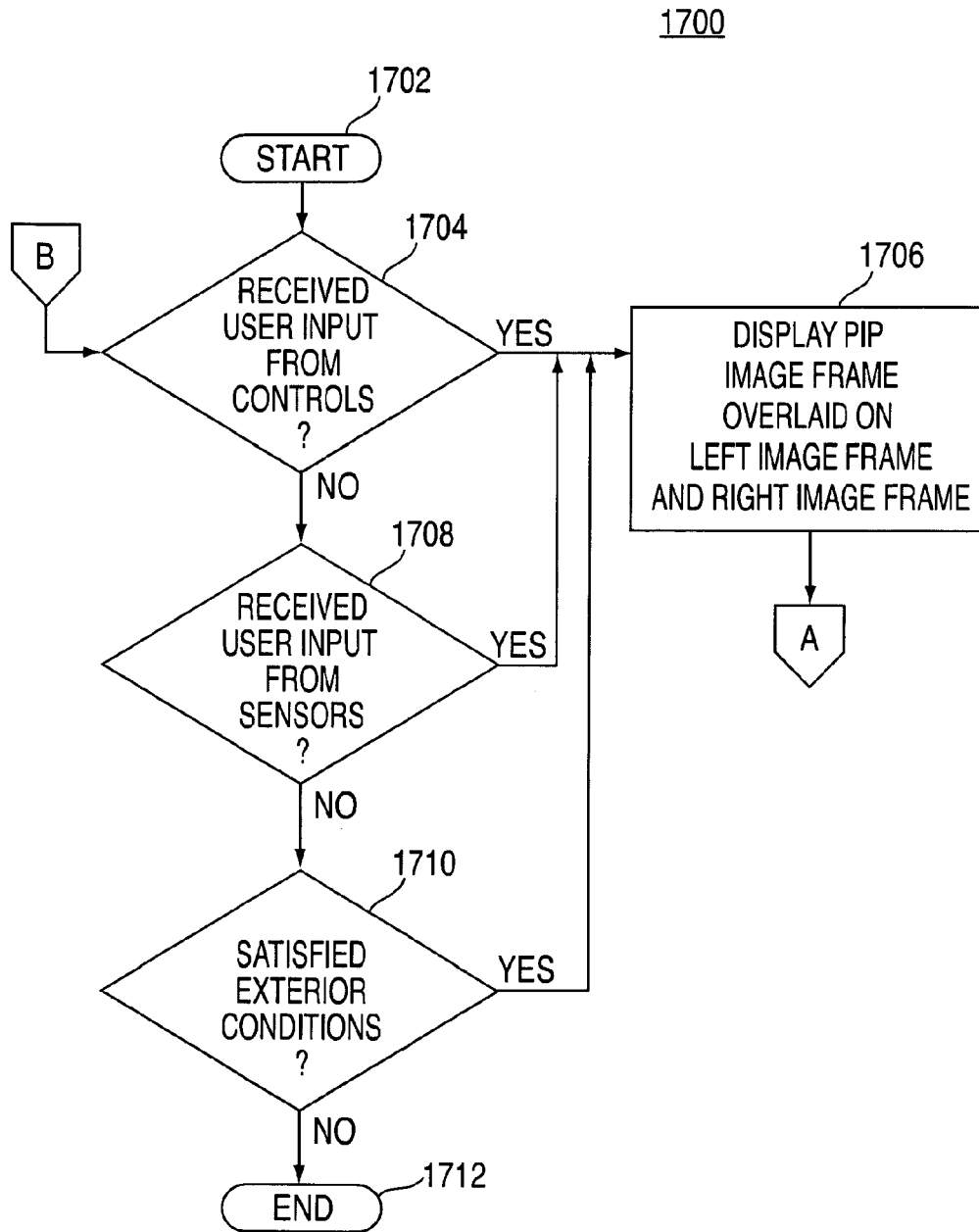
FIG. 17A
