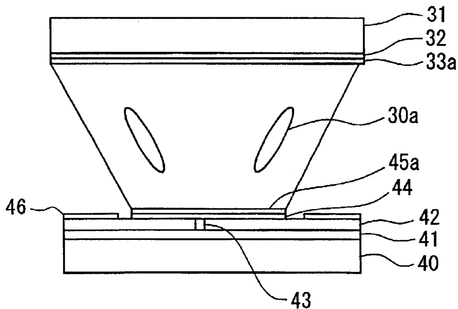
FIG. 21B
