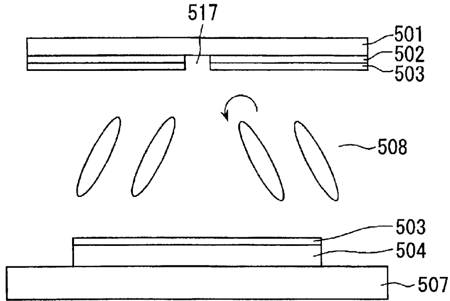
FIG. 44A
