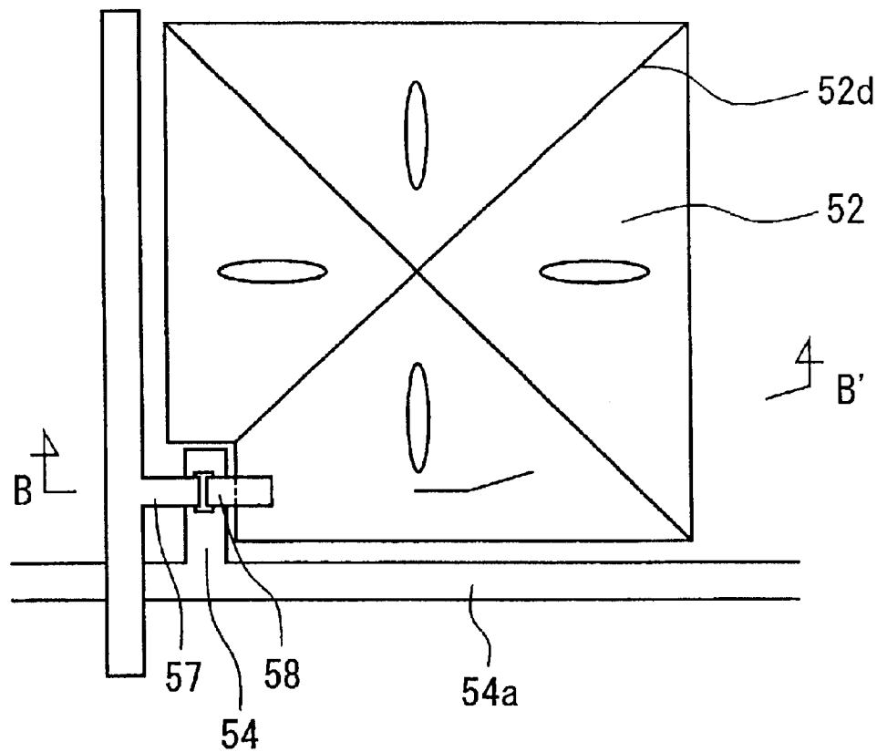
FIG. 24B
