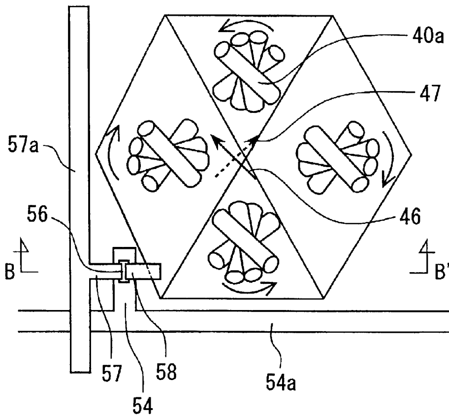
FIG. 25B
